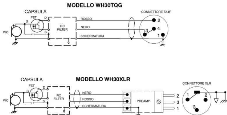
SCHEMI CIRCUITALI FIGURA 8
