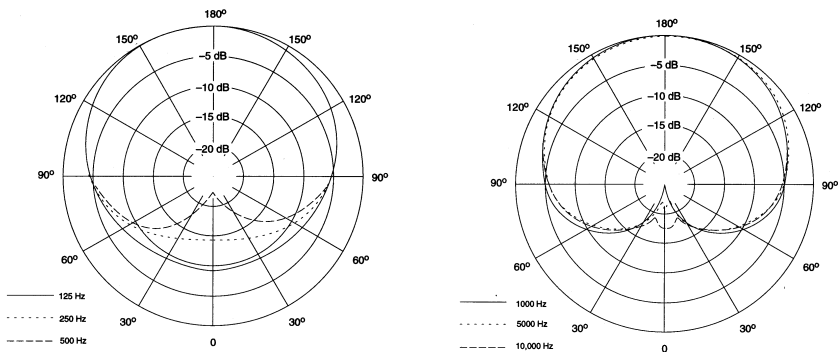
DIAGRAMMI POLARI TIPICI FIGURA 7
