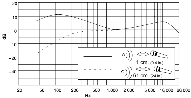
RISPOSTA IN FREQUENZA TIPICA FIGURA 6
