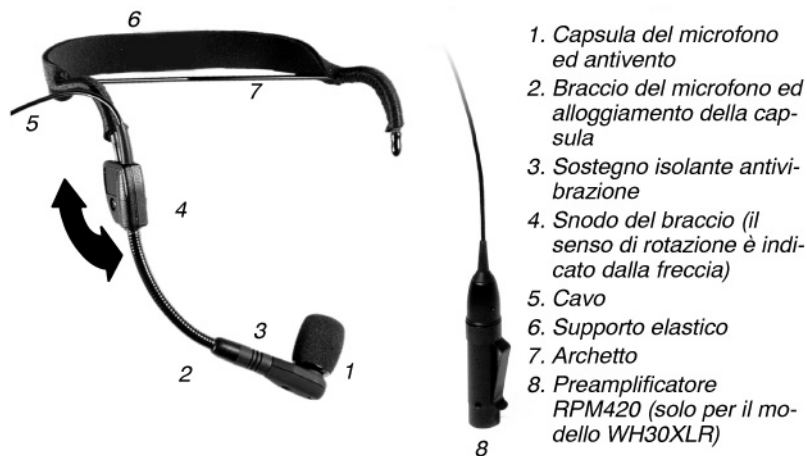
COMPONENTI DEL MICROFONO DOTATO DI GRUPPO CUFFIA WH30 FIGURA 1
