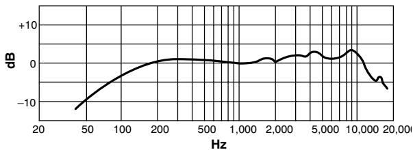
COURBE DE RÉPONSE EN FRÉQUENCE TYPIQUE FIGURE 6
